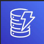
DynamoDB
