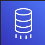
AWS DMS
