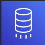
AWS SCT
