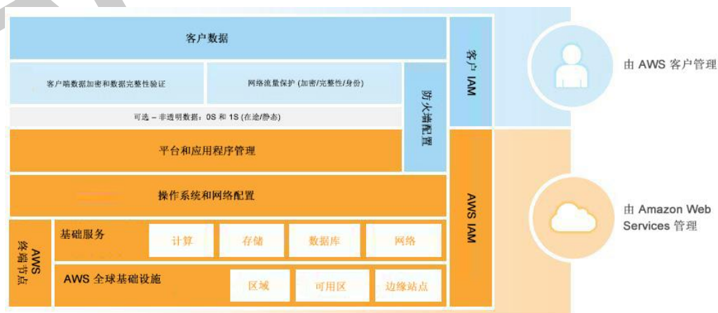
图 2：容器服务的责任共担模型
