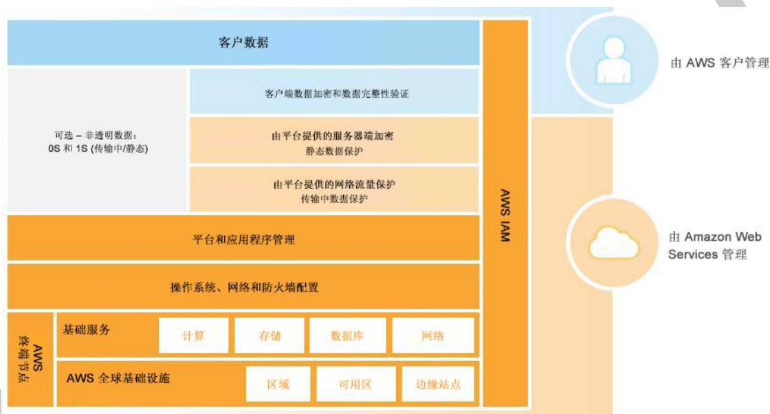
图 3：抽象服务的责任共担模型
